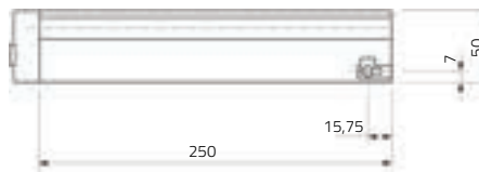
Zijaanzicht
