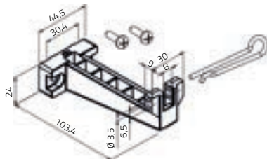
1731827: Valraamstoel
